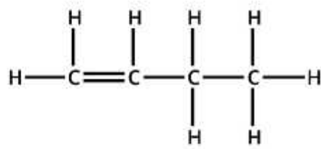
BUT-1-ENE
