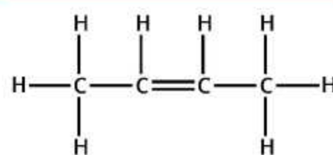
BUT-2-ENE
