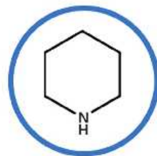
PIPERIDINE Azinane C_5H_{11}N
