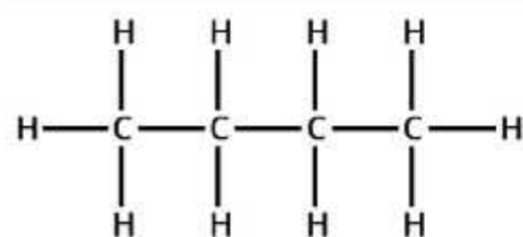
BUTANE
