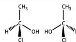
L: (S)-1-CHLOROETHANOL R: (R)-1-CHLOROETHANOL
